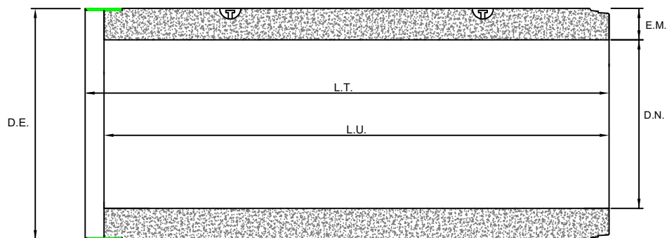
ANILLA DE ELEVACIÓN
