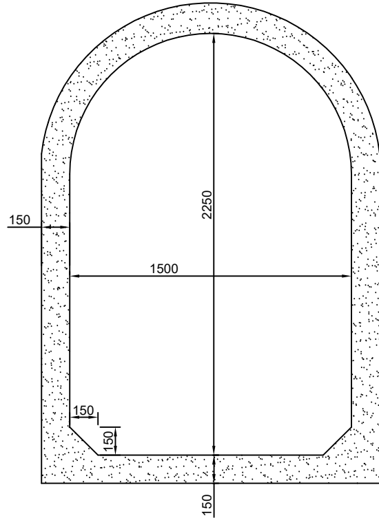
GALERÍA ABOVEDADA MACHIHEMRADA SIN ANDÉN TIPO III - AM
