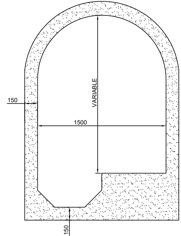
GALERÍA ABOVEDADA MACHIHEMRADA CON CUNA TRAPEZOIDAL
